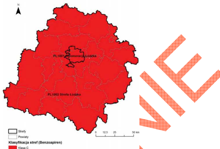
Rys. 18. Klasyfikacja stref w ocenie za rok 2019 dla benzo(a)pirenu
