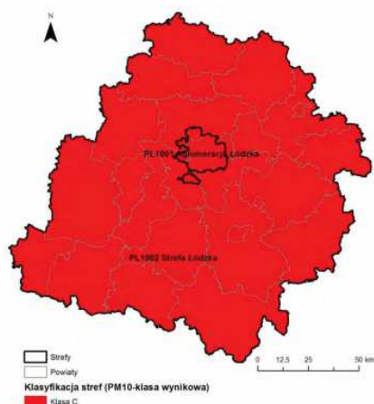
Rys. 13. Klasyfikacja stref w ocenie za rok 2019 dla pyłu PM10 (klasa wynikowa)
