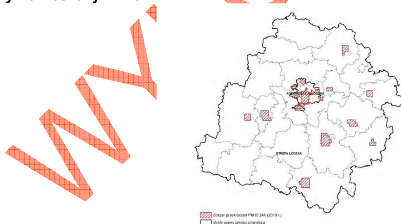
Rys. 11. Obszar przekroczeń dobowej wartości poziomu dopuszczalnego stężenia pyłu PM10 w województwie łódzkim w 2019 r.
