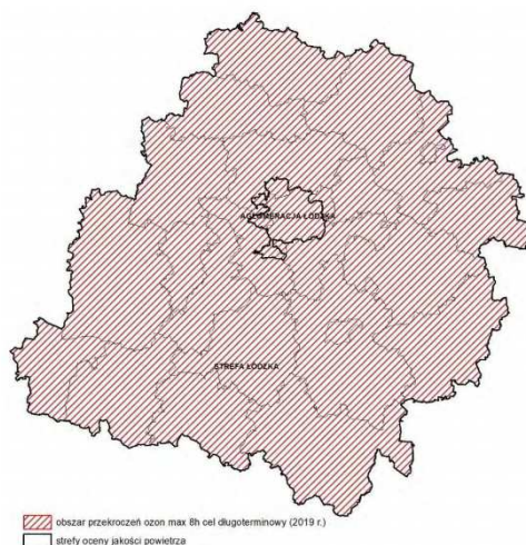
Rys. 21. Obszar przekroczeń wartości celu długoterminowego ozonu określonego ze względu na ochronę zdrowia (wartość 8-godz.) w województwie łódzkim w 2019 r.
