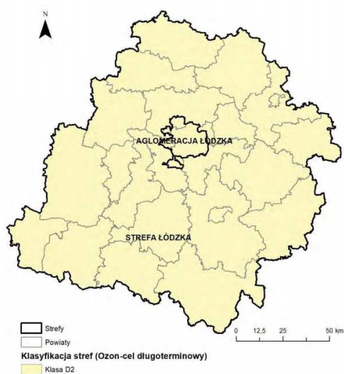
Rys.20. Klasyfikacja stref w ocenie za rok 2019 dla ozonu (poziom celu długoterminowego)
