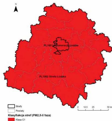
Rys. 17. Klasyfikacja stref w ocenie za rok 2019 dla pyłu PM 2,5 (faza II)
